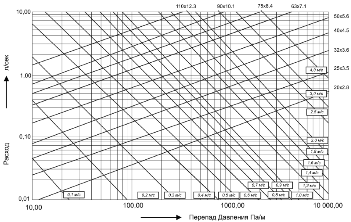
Номограмма потерь давления для труб РОСТерм FRP, армированных стекловолокном, SDR7,4 при температуре 20 °С
