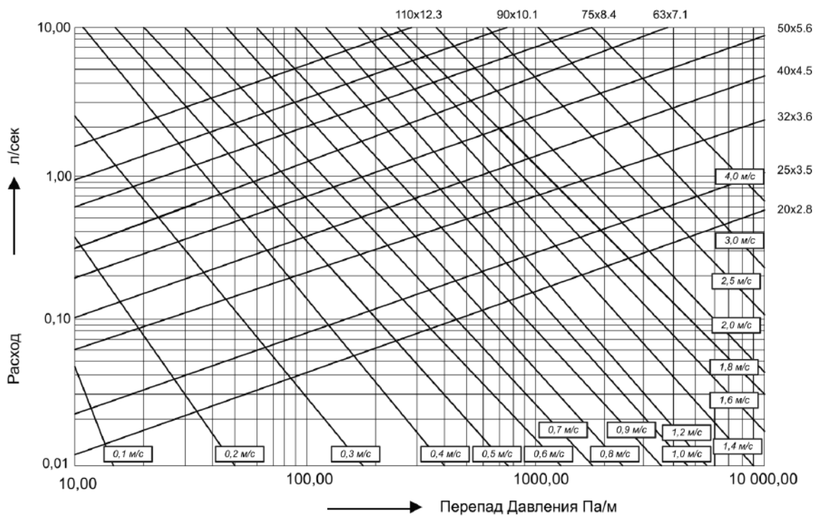
Номограмма потерь давления для труб РОСТерм FRP, армированных стекловолокном, SDR7,4 при температуре 60 °С
